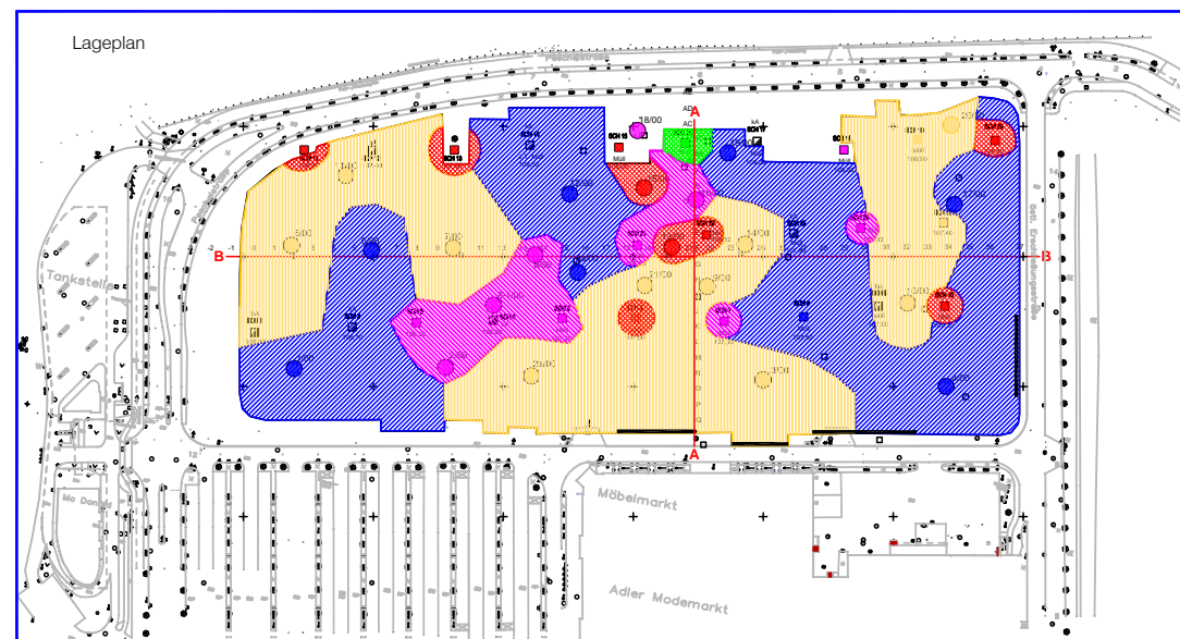
Unsortierter Aushub
